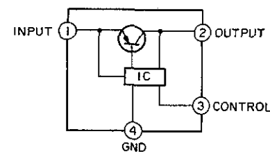
IC,PQ09R05
